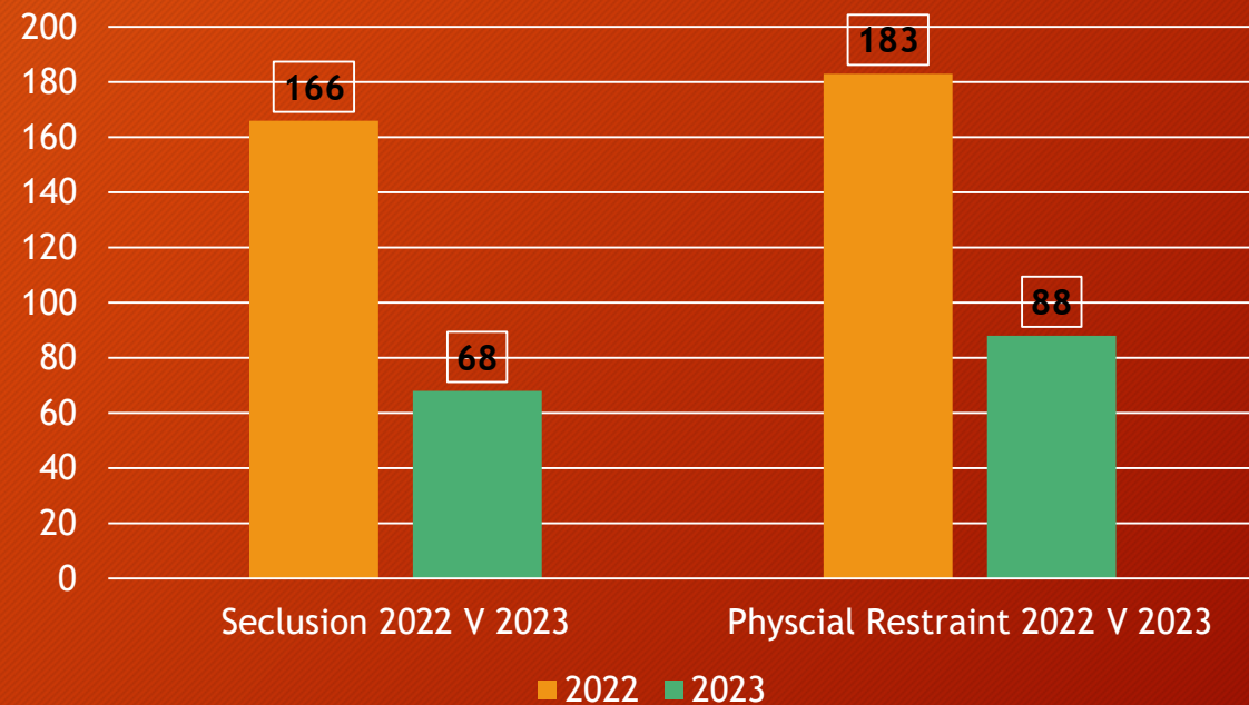
2022 V 2023 Data-DOP
